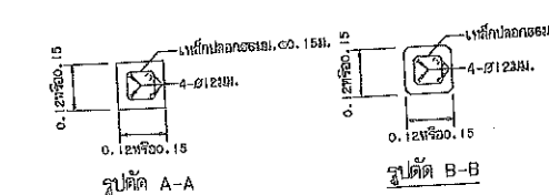
รูปตัดเสาป้าย
