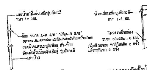
แสดงการติดตั้งป้ายบังคับ, ป้ายเตือน
