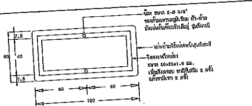
แสดงการยึดโครงป้ายโครงถัก น-1
